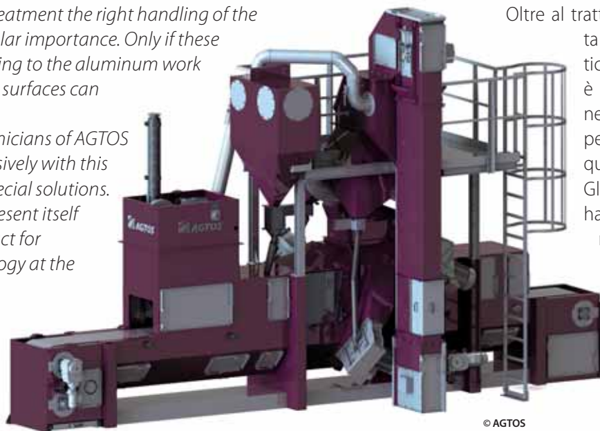
AGTOS-Wire mesh conveyor shot blast machine, Type BS. Granigliatrice con trasportatore a rete metallica AGTOS, tipo BS.
